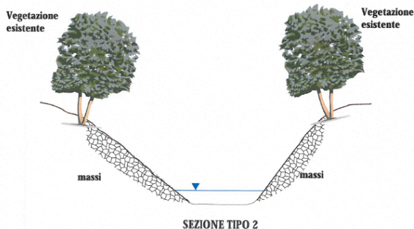
SEZIONE TIPO 2
