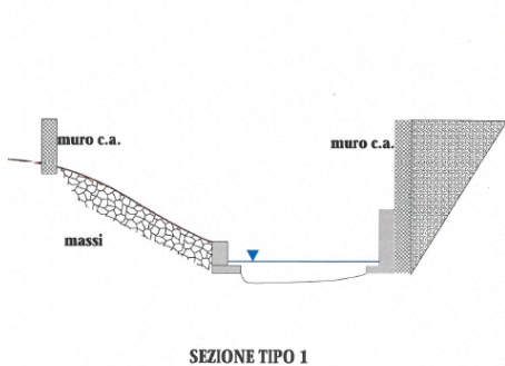
SEZIONE TIPO 1
